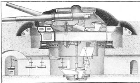
Schnitt durch den Panzerturm mit den zwei 28-cm SK/L 40 Kanonen
