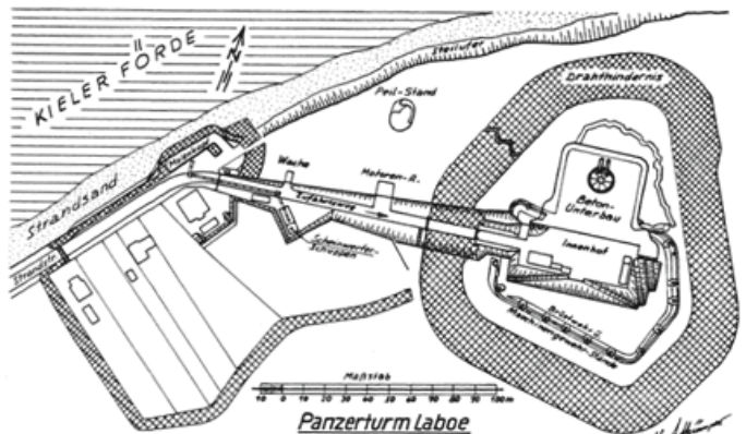
Panzerturm Laboe Bauzeit: 1899-1902 · Demontage u. Sprengung: 1919/20 Armierung: zwei 28-cm-Schiffskanonen in einem Panzerturm Der Beton-Unterbau hatte folgende Raumaufteilung: 1 Hohlraum für den Panzerturm, 2 Dampfkesselräume, 1 Maschinenraum, 1 Handpumpenraum, 2 Geschossräume, 2 Kartuschenräume, 5 Mannschalträume und 1 Küchenraum.
