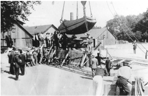
1901: Ein Schienenwagen auf dem Laboer Hafenplatz wird mit einem 49 Tonnen schweren Hartgusssegment für den Transport zum Panzerturm beladen
